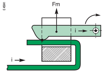
Пример отталкивания контактов
