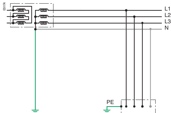
Система TT
