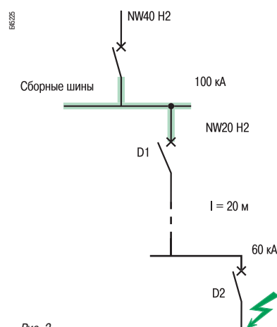
Рис. 2 Полная селективность
