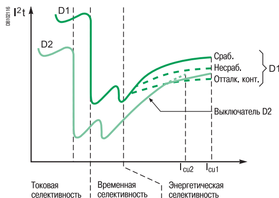
Селективность, усиленная каскадным соединением: кривые
