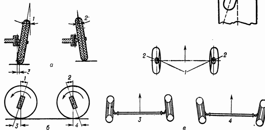
Рис. 55. Steering geometry геометрическая схема установки управляемых колёс.
