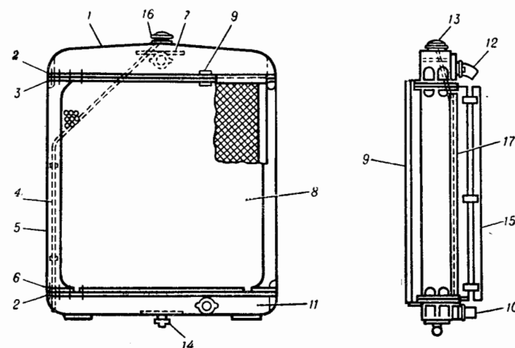
Рис. 27. Radiator радиатор.
