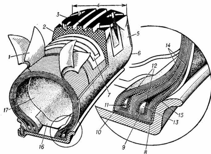
Рис. 57. Component parts of tire элементы шины.
