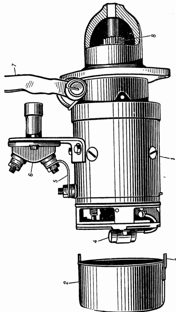
Рис. 111. Starter стартер. 1 — starter housing корпус стартера. 2 — end cover [горючая] крышка. 3 — starter clip защёлка крышки. 4 — capacitor конденсатор. 5 — starter-to-terminal connector соединитель стартера с пусковым переключателем. 6 — starter switch пусковой переключатель. 7 — shifting lever рычажок включения стартера. 8 — starter gear шестерня стартера.
