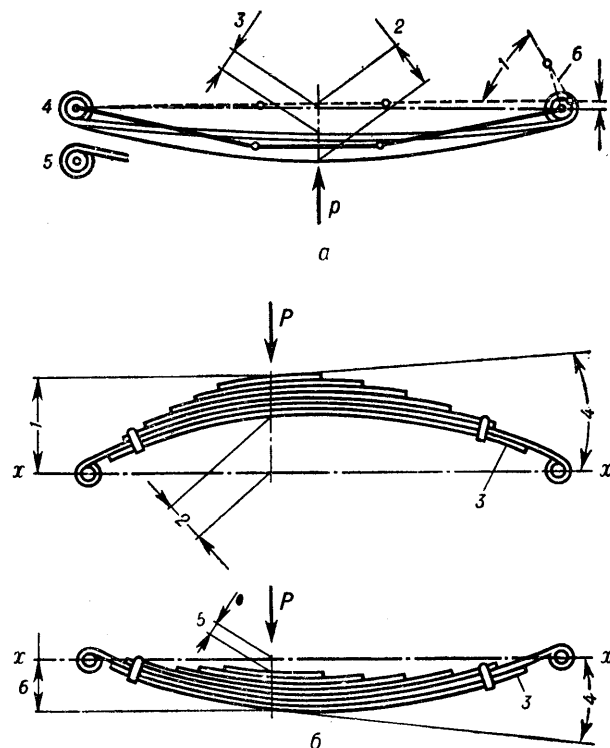
Рис. 48. Spring deflection деформация рессоры, прогиб рессоры.
