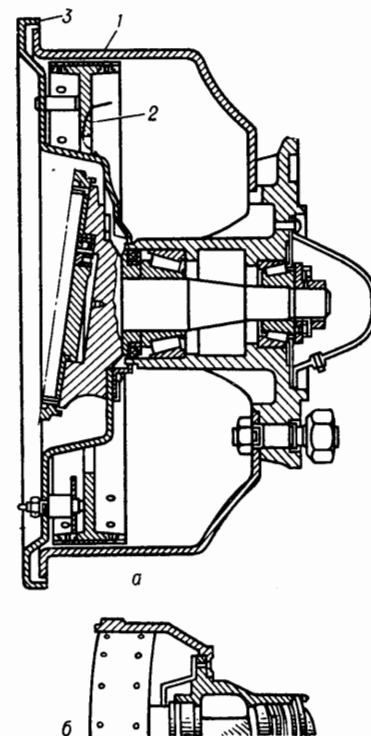
Рис. 67. Wheel brake колёсный тормоз. а — internal wheel brake колёсный тормоз с колодками внутри тормозного барабана. 1 — brake drum, wheel brake drum тормозной барабан. 2 — brake shoe, brake block тормозная колодка. 3 — brake anchor plate опорный диск тормозных колодок. б — outside-mounted brake тормоз, расположенный с внешней стороны колеса.
