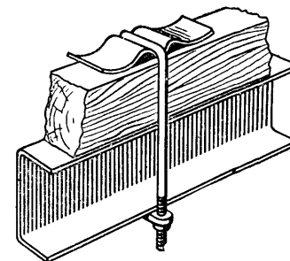
Рис. 81. Spring bearer plate пружинная прижимная пластина крепления (деталь кузова или платформы к раме).
