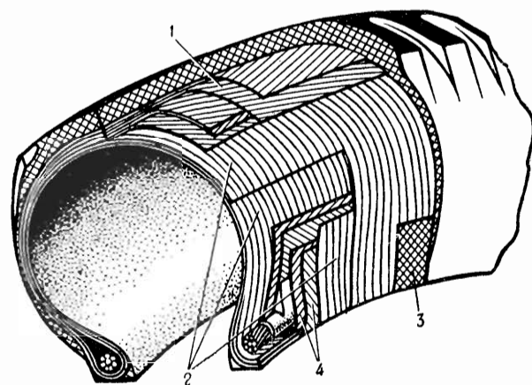
Рис. 60. Cross-biased tire шина с диагональным кордом. 1 — cross-biased casing ply слой диагонального каркаса. 2 — bead wire ring бортовое проволоочное кольцо. 3 — bead stiffener бортовой элемент жесткости.
