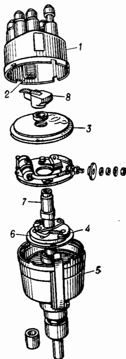
Рис. 30. Distributor распределитель. 1 — cap крышка. 2 — carbon brush угольная щётка. 3 — dust excluding plate пылезащитная пластина. 4 — automatic spark timer автоматический регулятор опережения зажигания. 5 — body корпус. 6 — plate пластина. 7 — cam кулачок прерывателя распределителя. 8 — rotating electrode вращающийся электрод.
