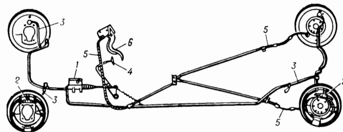
Рис. 71. Hydraulic foot brake and cable-operated hand brake тормоз с гидравлическим приводом от педали и ручной тормоз с тросовым приводом. 1 — brake master cylinder главный тормозной цилиндр. 2 — wheel cylinder, wheel-braking cylinder колёсный тормозной цилиндр. 3 — hydraulic brake hose шланг гидравлического тормозного привода. 4 — brake pedal тормозная педаль. 5 — brake cable трос тормоза. 6 — brake handle, brake hand lever рукоятка тормозного рычага.
