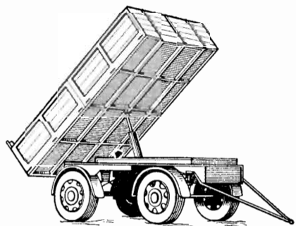
Рис. 94. End-tip trailer прицеп-самосвал с задней разгрузкой.
