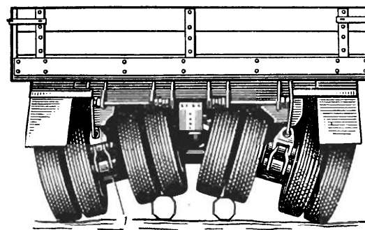
Рис. 40. Oscillating axle 1 — качающаяся ось.
