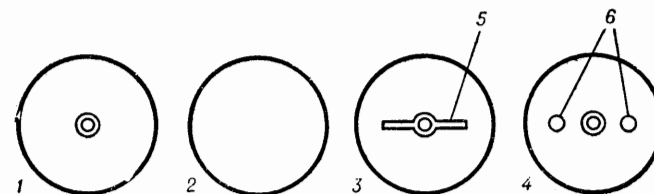
Рис. 16. Types of valve heads типы тарелок [головок] клапанов.
