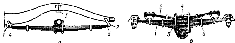
Рис. 47. Leaf spring attachment крепление листовой рессоры.
