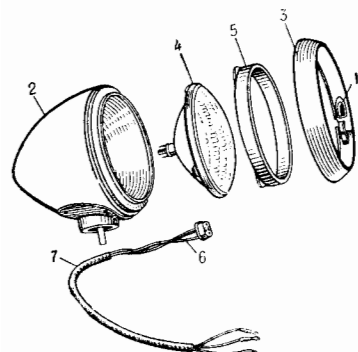
Рис. 29. Head lamp parts детали фары. 1 — clip пружинный держатель. 2 — body корпус. 3 — moulding наружный ободок. 4 — sealed beam unit оптический элемент. 5 — sealed beam unit retaining ring внутренний [установочный] ободок оптического элемента. 6 — wiring assembly пучок проводов. 7 — wiring loom гибкая изолирующая трубка для проводов.
