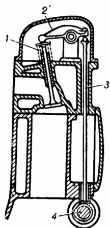
Рис. 19. Valve-(actuating) gear клапанный привод, клапанный механизм.
