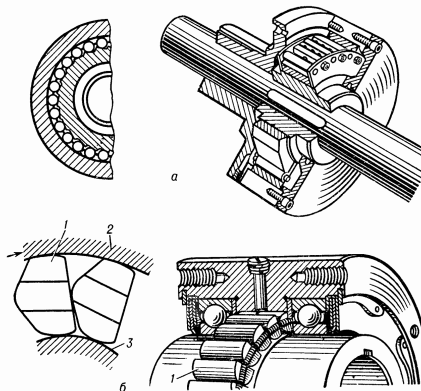
Рис. 37. Free-wheeling clutch, overrunning clutch муфта свободного хода. a — roller-type overrunning c., free-wheeling roller c., overrunning roller c., roller-type free-wheeling c. with polygon cam муфта свободного хода, работающая по принципу заклинивания цилиндрических роликов между цилиндрическим и профилированным кольцами. б — sprag-type overrunning c., free-wheeling sprag c., overrunning sprag c., sprag c. муфта свободного хода, работающая по принципу заклинивания брусьев между цилиндрическими наружным и внутренним кольцами. 1 — sprag расклинивающий сухарь. 2 — outer race наружное кольцо. 3 — inner race внутреннее кольцо.
