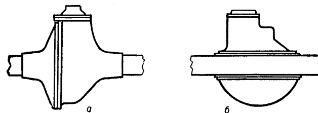
Рис. 42. Driving axle housing, driving axle case картер ведущего моста. a — split housing, split case разъёмный картер. b — banjo housing, one-piece housing, banjo case неразъёмный картер.
