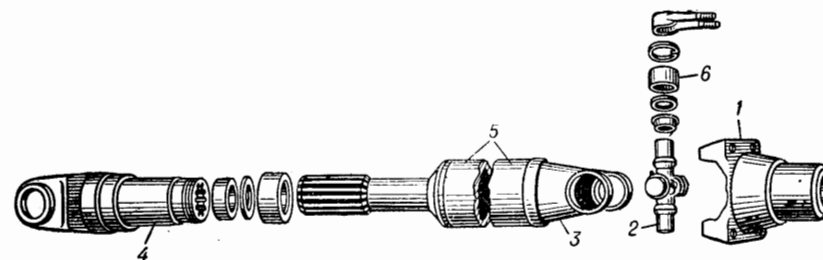
Рис. 38. Universal-joint drive, cardan drive карданная передача, карданный привод. 1 — universal-joint flange фланец крепления кардана. 2 — universal-joint center cross, trunnion cross крестовина кардана. 3 — universal-joint fork, universal-joint yoke вилка кардана. 4 — universal-joint slip yoke скользящая вилка кардана. 5 — universal-joint shaft tube, propeller-shaft tube труба карданного вала. 6 — needle bearing with closed end игольчатый роликовый подшипник с закрытым торцом.
