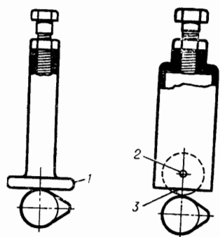
Рис. 18. Mushroom and roller-type valve lifters толкатели клапана: грибовидный (слева) и с роликом (справа).
