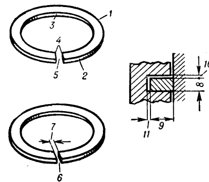
Рис. 6. Piston ring поршневое кольцо.
