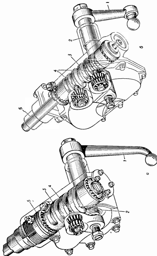
Рис. 63. Cam-and-lever steering gear, peg-and-worm steering gear рулевой механизм с червяком и кривошипом.
