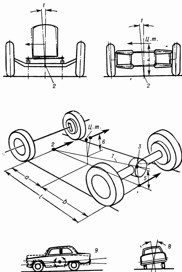
Рис. 52. Rolling крен (автомобиля).
