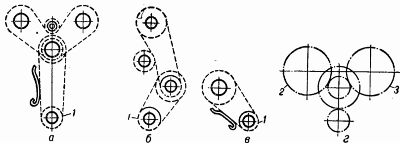
Рис. 20. Types of camshaft drives типы приводов распределительных валов.
