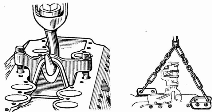
Рис. 100. Engine lifting fixture скоба для подъема двигателя.
