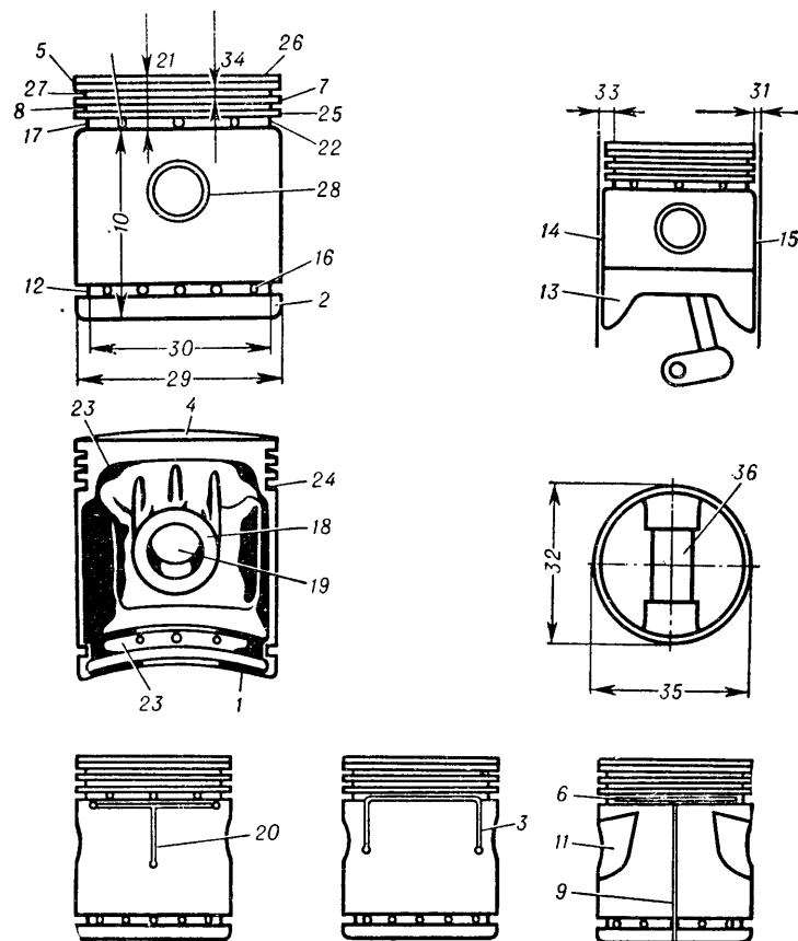
Рис. 3. Piston поршень.
