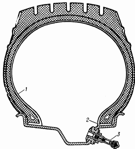
Рис. 61. Tubeless tire бескамерная шина.
