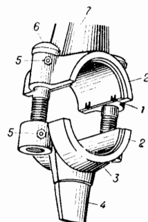
Рис. 13. Connecting rod big end большая головка шатуна.
