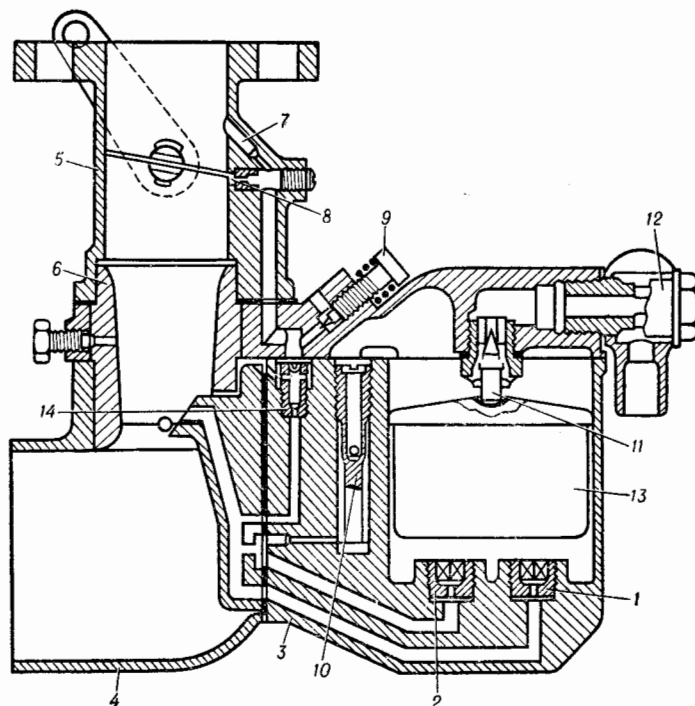
Рис. 26. Carburetor карбюратор.
