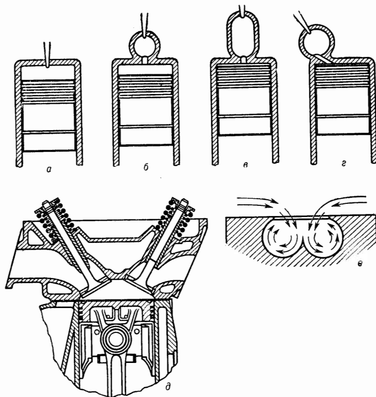
Рис. 22. Types of combustion chambers типы камер сгорания.
