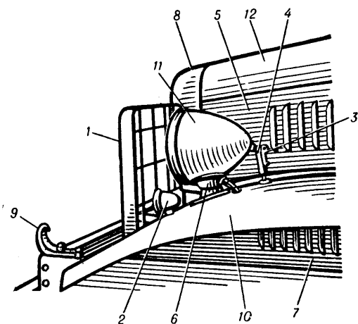
Рис. 82. Hood and fenders капот и крылья. 1 — brush guard защитная решётка фары. 2 — black-out marker lamp габаритный фонарь со светомаскировкой. 3 — hood catch bracket гнездо запора капота. 4 — hood catch замок [запор] капота. 5 — hood side panel боковина капота, боковая панель капота. 6 — lamp bracket, lamp carrier кронштейн фары. 7 — mud shield брызговик. 8 — radiator shell облицовка радиатора. 9 — towing hook буксирный крюк. 10 — front fender, front wing переднее крыло. 11 — head lamp фара. 12 — hood капот.
