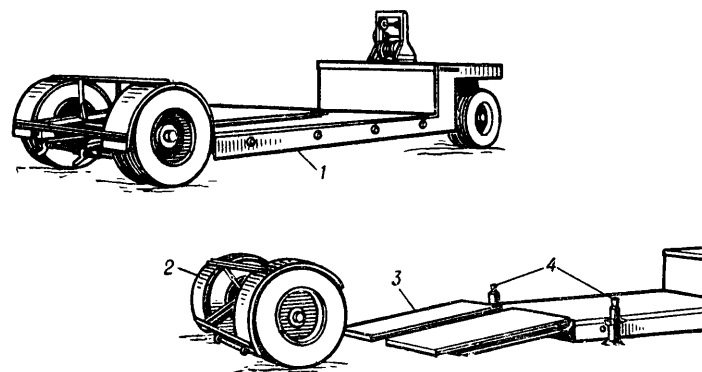
Рис. 89. 1 — Trailer with withdrawable rear axle, trailer with detachable rear axle прицеп со съёмной задней осью. 2 — withdrawable rear axle съёмный задний мост. 3 — loading ramp погружной наклонный трап. 4 — jack домкрат.
