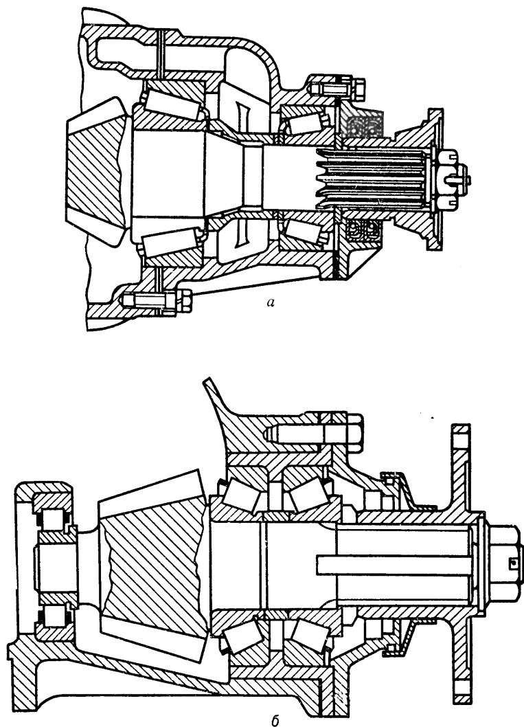
Рис. 39. Axle drive pinion ведущая шестерня главной передачи. a — overhung p. консольно-смонтированная ведущая шестерня. b — straddle-mounted p. ведущая шестерня, смонтированная между двумя опорами.
