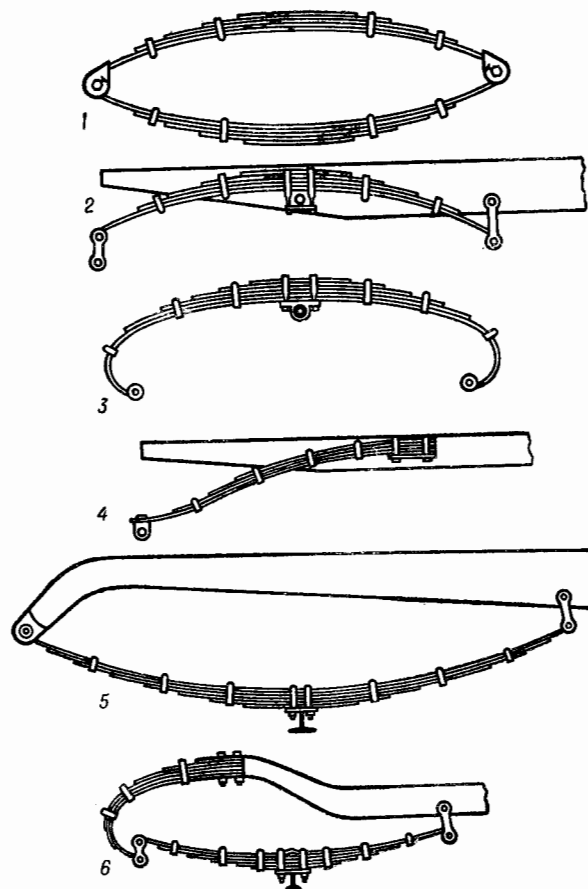
Рис. 46. Laminated spring, leaf spring листовая рессора.
