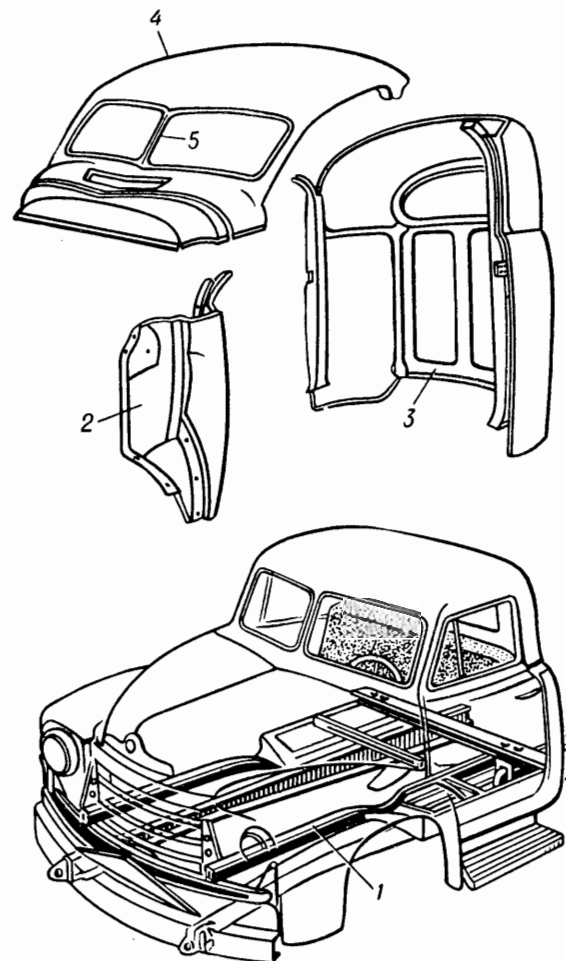
Рис. 78. Parts of cab body детали кабины.
