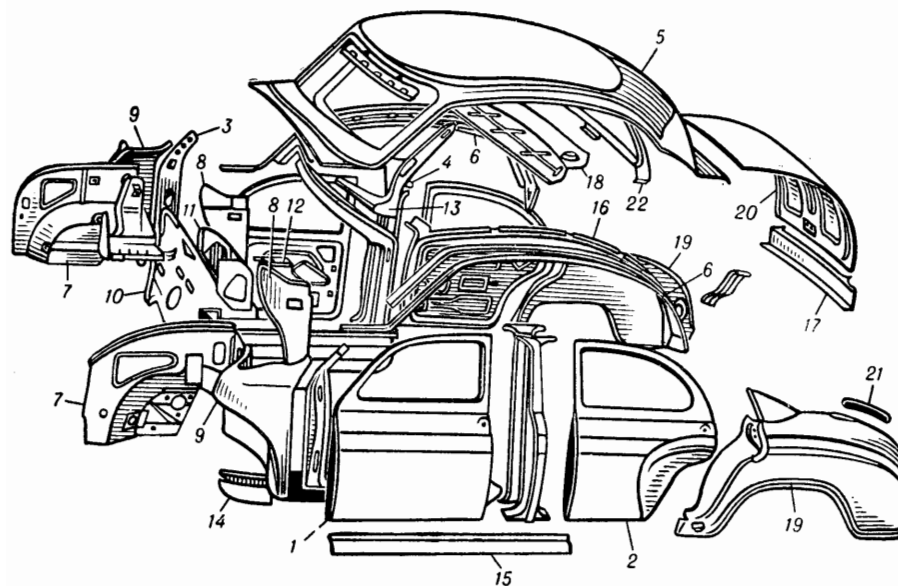
Рис. 76. Parts of car body детали кузова легкового автомобиля.
