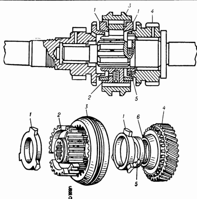
Рис. 35. Synchro-mesh unit, synchronizing device синхронизатор. 1 — block ring, blocking ring блокирующее кольцо. 2 — sliding hub скользящая ступица. 3 — synchronizer sleeve, synchronizing sleeve обойма синхронизатора. 4 — transmission gear шестерня коробки передач. 5 — locking ring замковое [стопорное] кольцо. 6 — synchronizing cone синхронизирующий конус.
