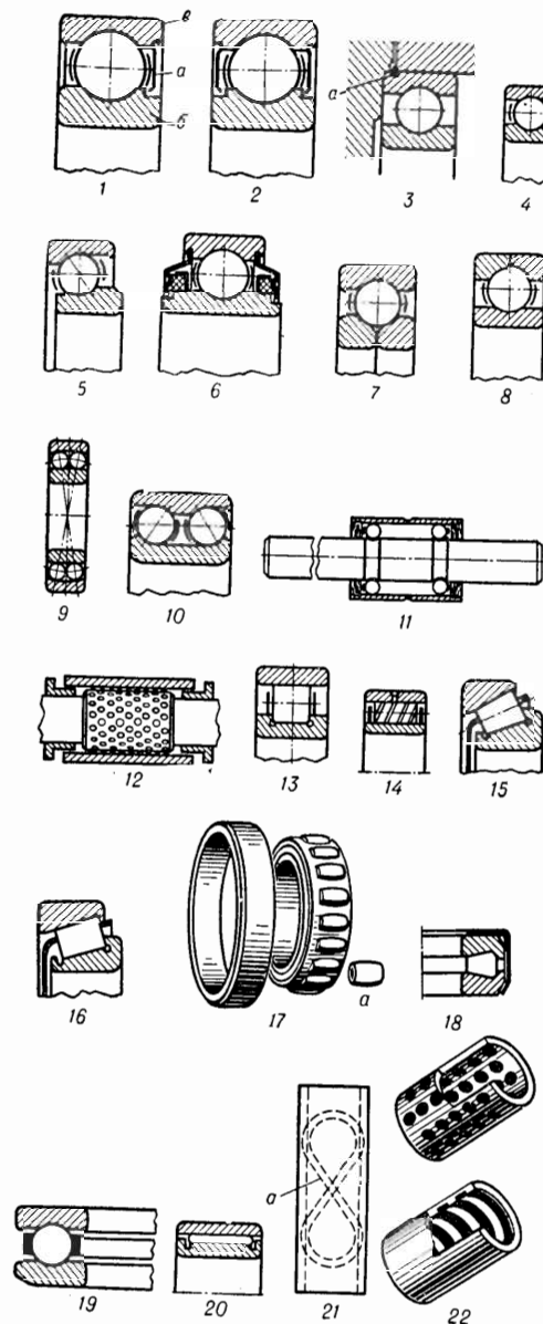
Рис. 96. Types of bearings типы подшипников.
