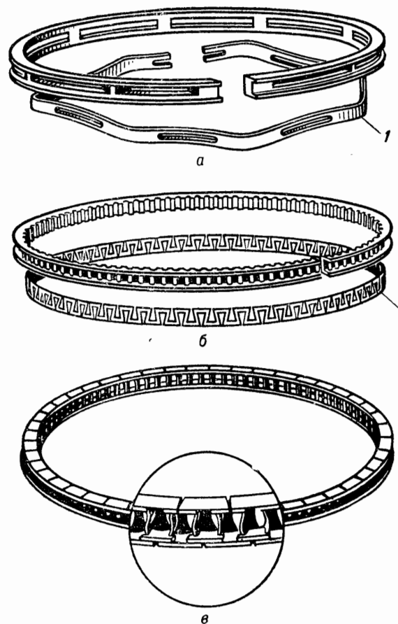
Рис. 11. Conformable oil piston ring, flexible oil piston ring, flexline oil piston ring маслоъемное поршневое кольцо с повышенной приспособляемостью к стенкам цилиндра.
