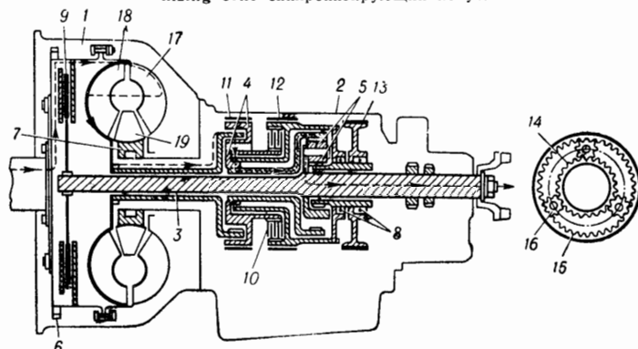
Рис. 36. Torque converter with planetary gearbox гидротрансформатор с планетарной коробкой передач. 1 — torque converter гидротрансформатор. 2 — planetary gearbox, planetary transmission планетарная коробка передач. 3 — main shaft главный [вторичный] вал. 4—5 — planetary gearset планетарный комплект (коробки передач). 6 — flywheel starter gear зубчатый венец маховика. 7—8 — free-wheel(ing) unit, free-wheel mechanism механизм свободного хода. 9 — direct-drive clutch, direct-driving clutch муфта включения прямой передачи. 10 — multi-disk clutch, multiplate clutch многодисковое сцепление. 11—13 — band brake ленточный тормоз. 14 — sun gear, sun wheel солнечная [центральная] шестерня планетарной передачи. 15 — ring gear зубчатое колесо с внутренним зацеплением. 16 — planet gear, planet(ary) pinion сателлит планетарной передачи. 17 — impeller насосное колесо. 18 — turbine турбинное колесо. 19 — stator статор.
