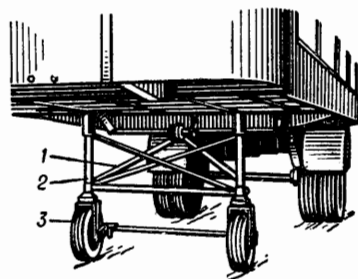
Рис. 95. Jockey wheel откидное опорное колесо.
