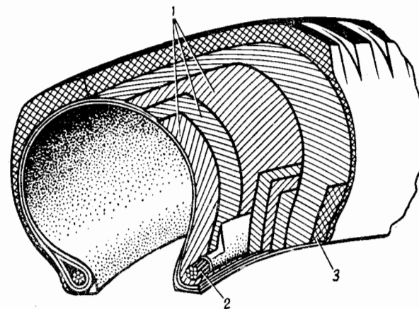
Рис. 59. Radial-ply tire шина с радиальным кордом.
