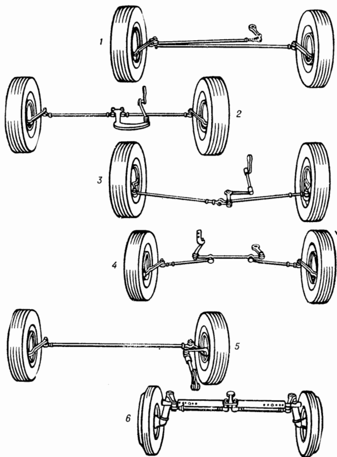
Рис. 66. Steering linkage nomenclature номенклатура рулевых приводов. 1 — cross steering linkage привод с поперечной тягой. 2 — center arm steering linkage привод с центральным рычагом (при нерегулируемой коле). 3 — Haltenberger linkage ahead of axle привод с центральным рычагом и трапецией расположенной впереди передней оси. 4 — parallellogram steering linkage привод с параллелограммными поперечными тягами. 5 — fore-aft-and-cross steering linkage привод с продольной и поперечной тягами. 6 — center-arm steering linkage привод с центральным рычагом (при регулируемой коле),
