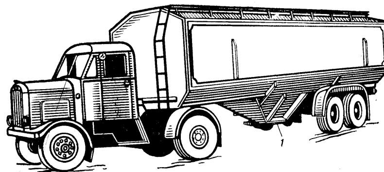
Рис. 84. Grain hopper body бункерный кузов для перевозки зерна. 1 — bottom discharge разгрузка через дно, разгрузка снизу.
