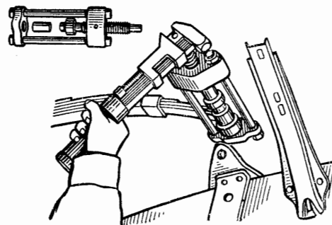
Рис. 103. Spring-hanger bushing replacer приспособление для замены втулок в ушках рессоры.
