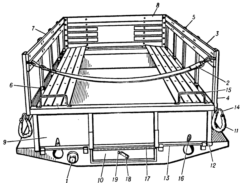
Рис. 79. Parts of platform body детали кузова-платформы.
