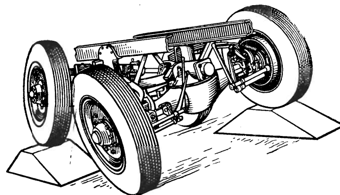
Рис. 41. Four-wheel drive bogie тележка с четырьмя ведущими колёсами.
