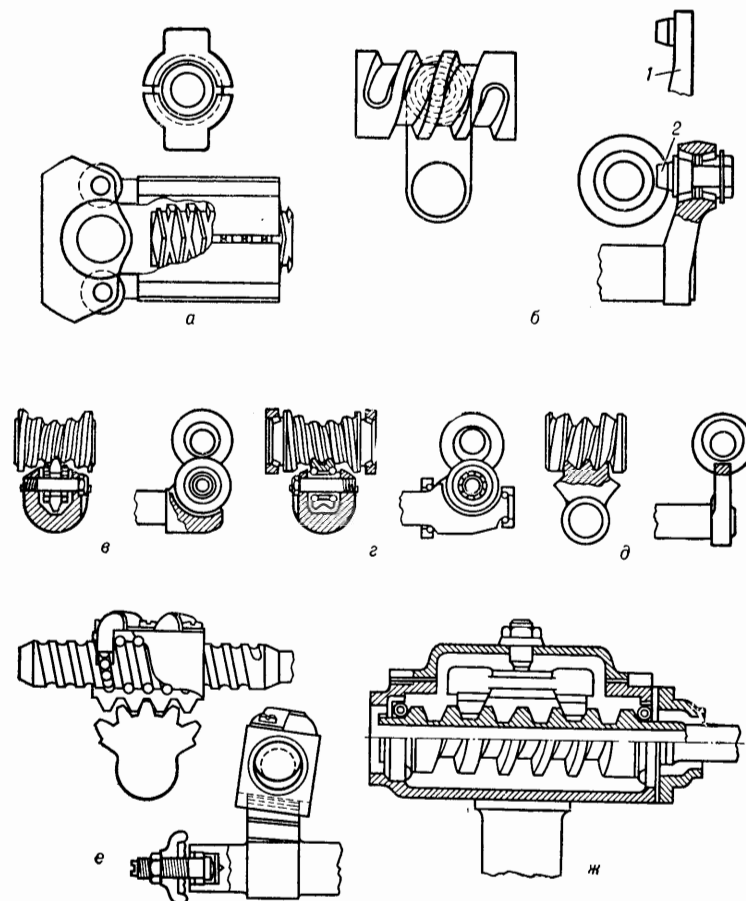
Рис. 62. Steering gear nomenclature номенклатура рулевых механизмов. а — worm-and-nut s. g., screw-and-nut s. g. рулевой механизм с винтом и гайкой; worm-and-double-nut s. g., screw-and-double-nut s. g. рулевой механизм с винтом и разрезной гайкой. б — cam-and-lever s. g., peg-and-worm s. g., worm-and-lever s. g. рулевой механизм с червяком и кривошипом. 1 — with fixed stud с закреплённым шипом. 2 — with roller stud с вращающимся шипом. в и г — worm-and-single-roller s. g., cam-and-roller s. g. рулевой механизм с червяком и роликом. в — worm-and-single-roller s. g., cam-and-single-roller s. g. рулевой механизм с червяком и одинарным роликом. г — worm-and-double-roller s. g., worm-and-twin-roller s. g., cam-and-double-roller s. g., cam-and-twin-roller s. g. рулевой механизм с червяком и двойным роликом. д — worm-and-sector s. g. рулевой механизм с червяком и сектором. е — circulating ball-and-nut s. g., ball bearing nut s. g., recirculating ball-and-nut s. g. рулевой механизм с гайкой и сектором. ж — cam-and-twin-lever s. g., worm-and-twin-lever s. g. рулевой механизм с червяком и двойным кривошипом.
