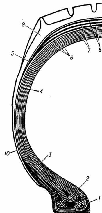
Рис. 58. Component parts of tire элементы шины.
