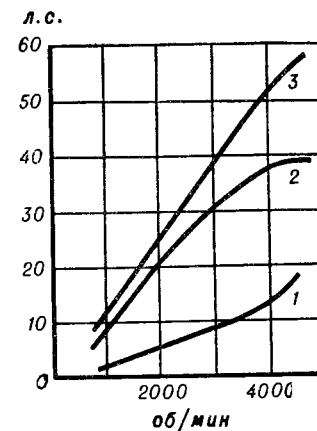
Рис. 1. Power curves of engine кривые мощности двигателя.
