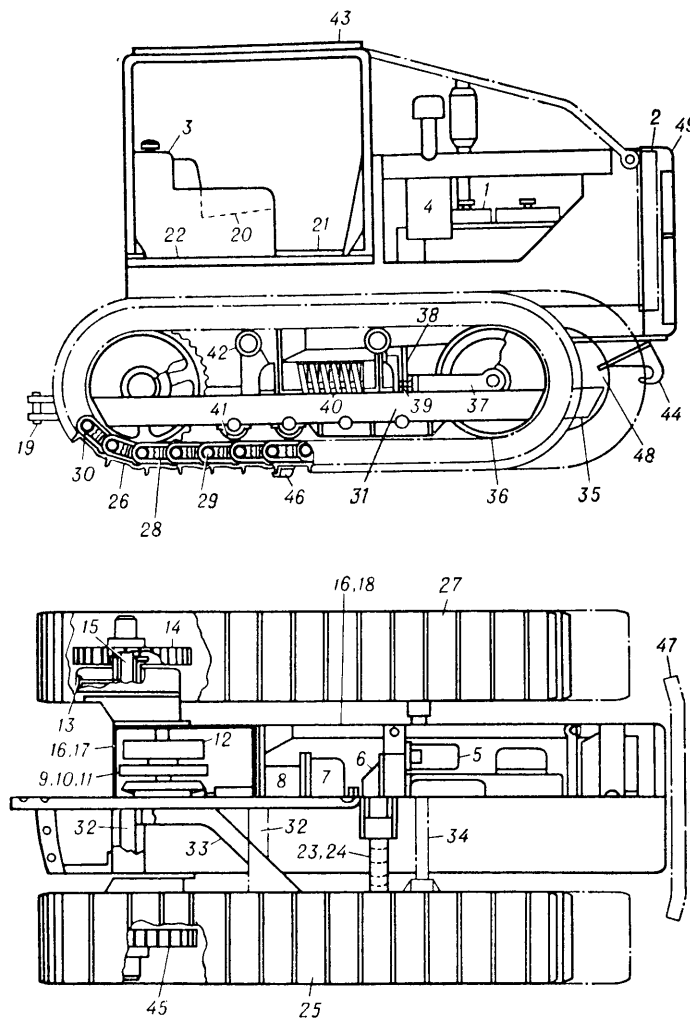
Рис. 109. Caterpillar tractor гусеничный трактор.
