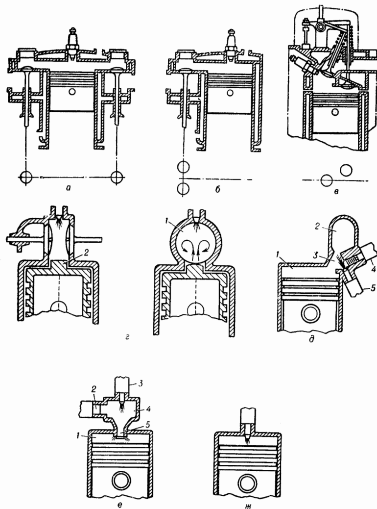
Рис. 21. Various forms of cylinder heads различные виды головок цилиндров (кругами под рисунками а, б, в схематически показано расположение клапанов).
