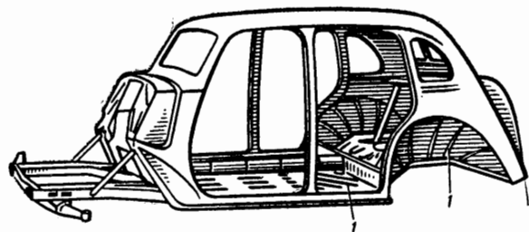
Рис. 73. Integral chassis and body construction конструкция шасси с несущим кузовом. 1 — ribbing выштампованные ребра.
