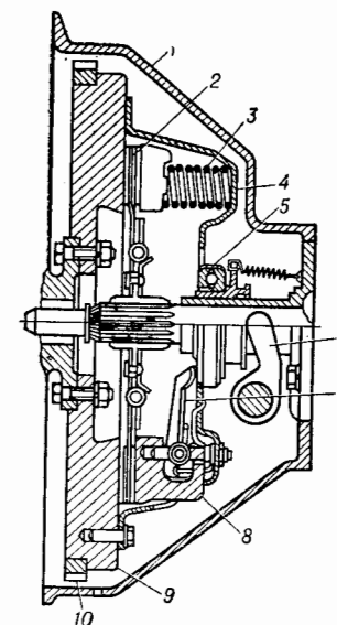
Рис. 31. Clutch сцепление. 1 — housing картер. 2 — driven plate, driven disk ведомый диск. 3 — pressure spring нажимная пружина. 4 — cover plate, back plate опорный диск. 5 — throw-out bearing, clutch release bearing подшипник выключения сцепления. 6 — bearing release lever рычаг [отводка] выжимного подшипника. 7 — release lever рычаг выключения. 8 — pressure plate нажимной диск. 9 — flywheel маховик. 10 — flywheel (ring) gear, flywheel starter gear зубчатый венец маховика.
