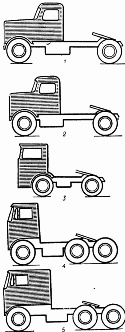
Рис. 110. Types of tractors типы тягачей. 1 — conventional tractor тягач обычной компоновки. 2 — short conventional tractor укороченный тягач обычной компоновки. 3 — tilt cab tractor тягач с откидной кабиной. 4 — high tilt cab tractor тягач с высокорасположенной откидной кабиной. 5 — high tilt cab tractor with sleeper тягач с высокорасположенной откидной кабиной со спальным местом.
